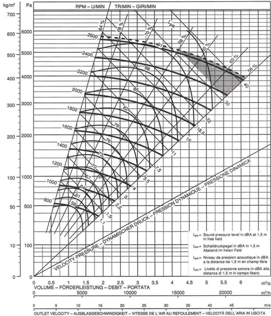
PA 610 Girante \phi 609 Bocca aspirante \phi 450 - Bocca premente 336 x 375
