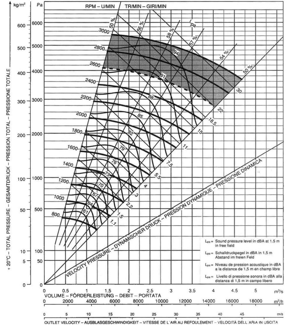
PA 550 Girante \phi 548 Bocca aspirante \phi 400 - Bocca premente 305 x 348
