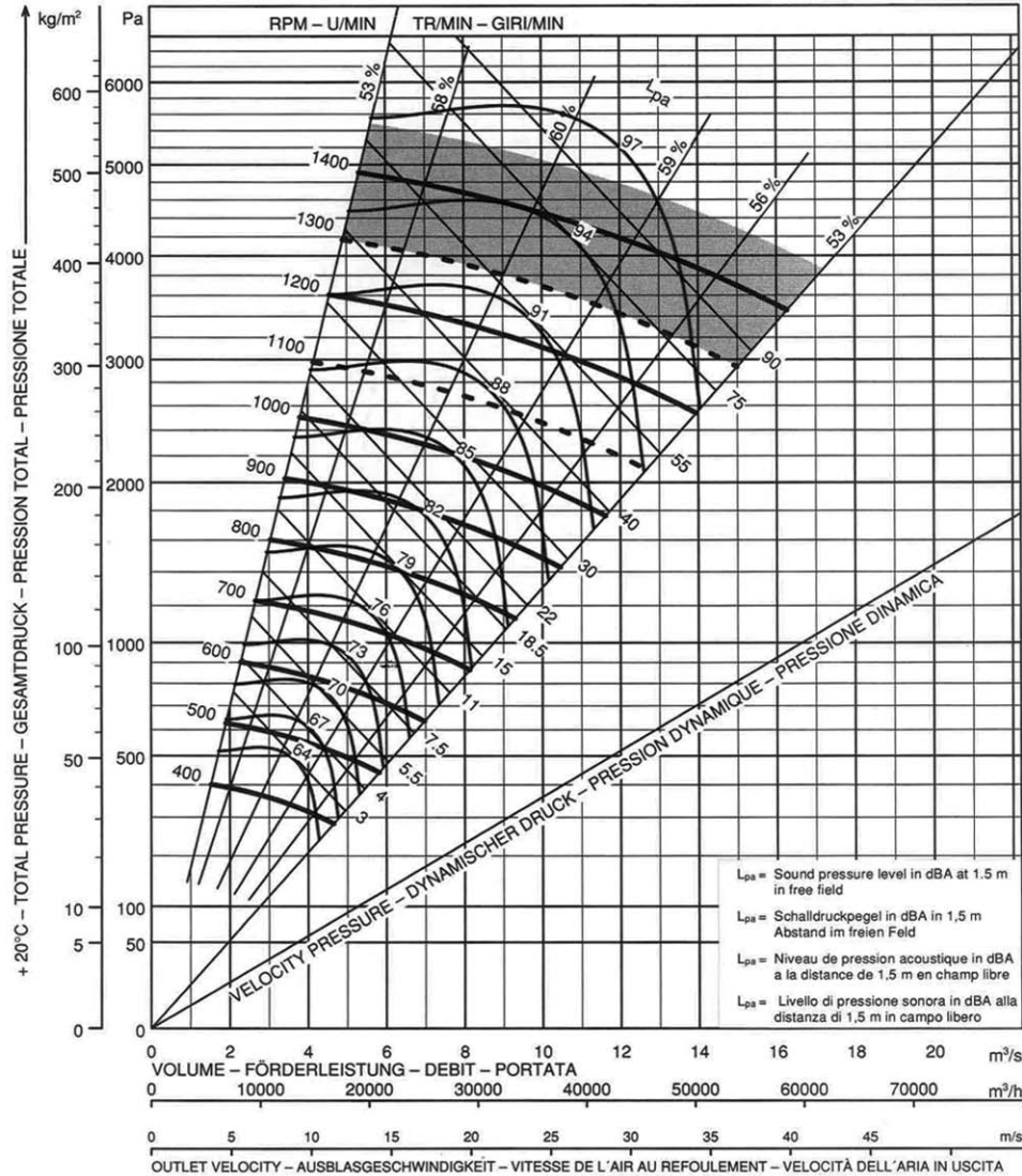
PA 1100 Girante \phi 1096 Bocca aspirante \phi 750 - Bocca premente 600 x 670
