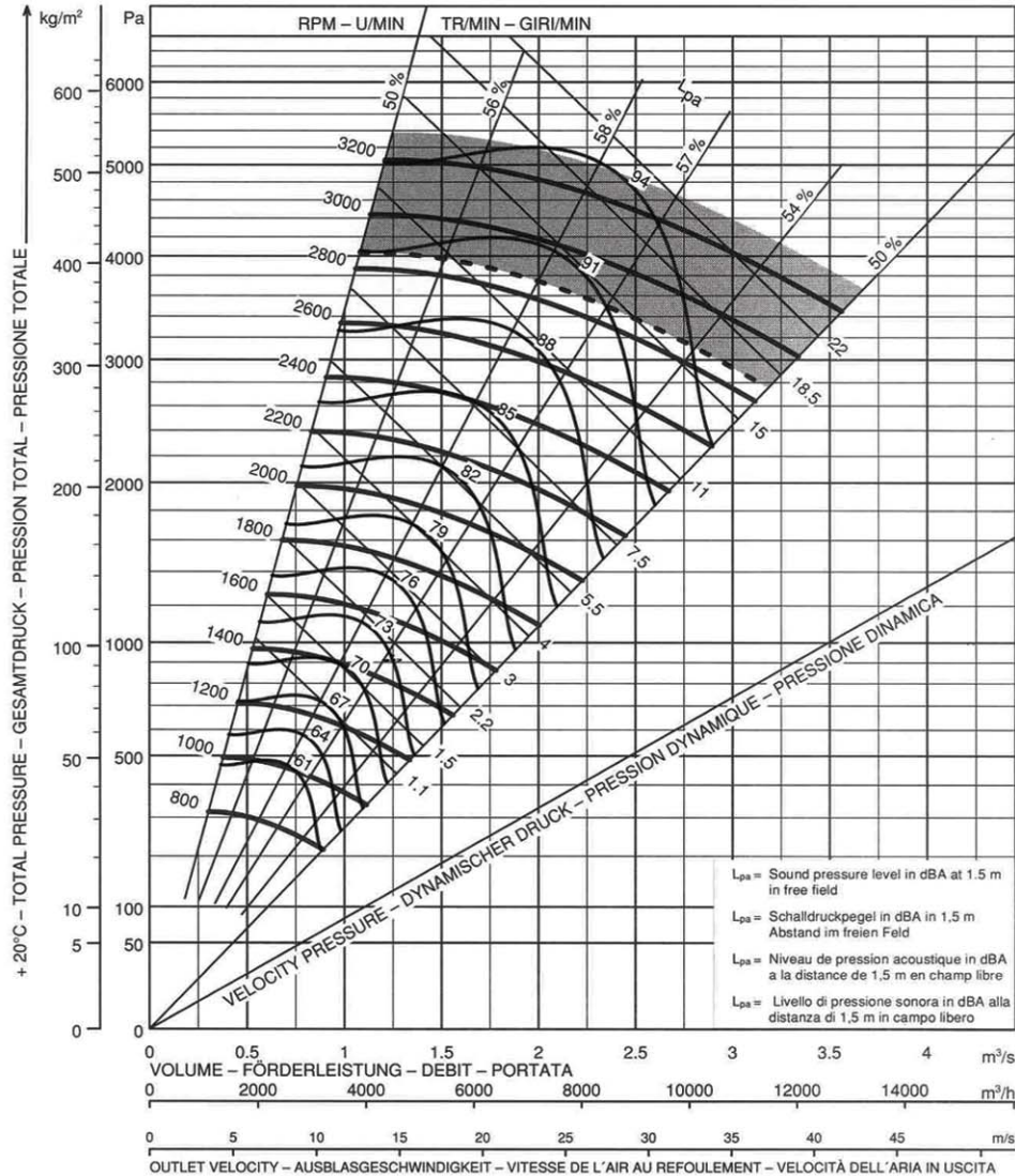
PA 500 Girante \phi 500 Bocca aspirante \phi 350 - Bocca premente 272 x 300
