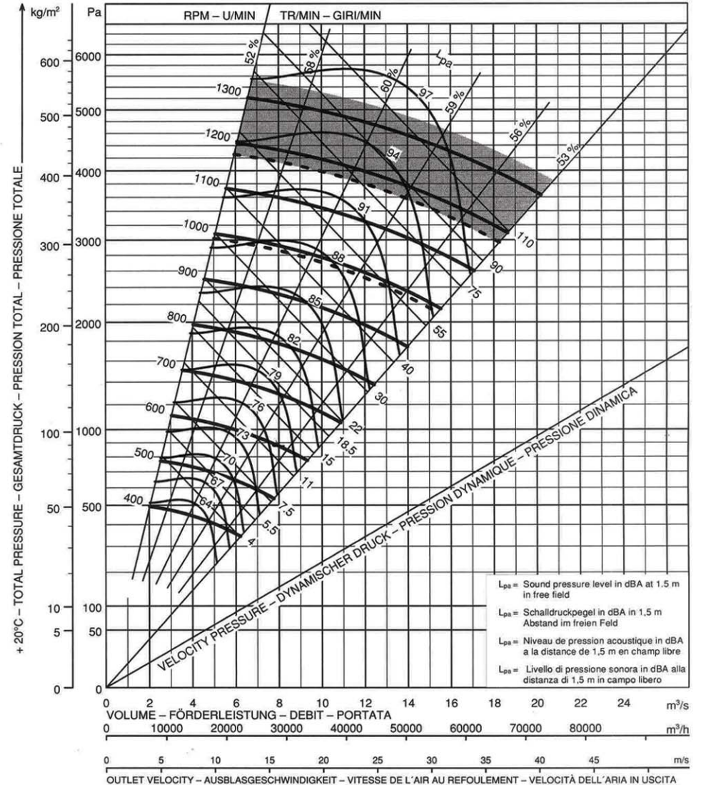
PA 1200 Girante \phi 1219 Bocca aspirante \phi 850 - Bocca premente 660 x 750
