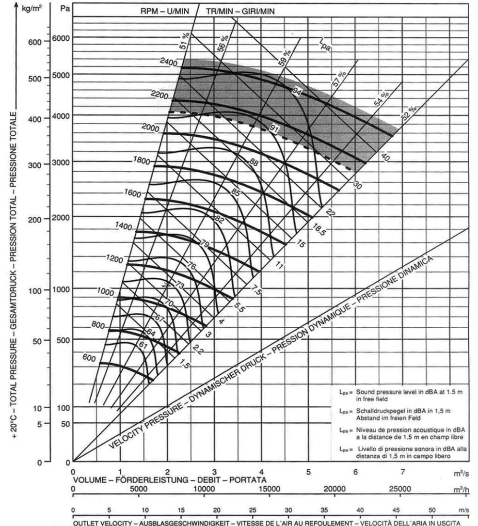
PA 670 Girante \phi 671 Bocca aspirante \phi 500 - Bocca premente 370 x 415
